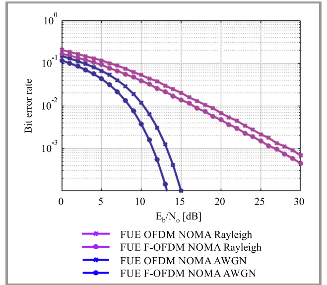
Fig. 10. BER performance of FUE in downlink F-OFDM NOMA in AWGN and over the Rayleigh channel.
