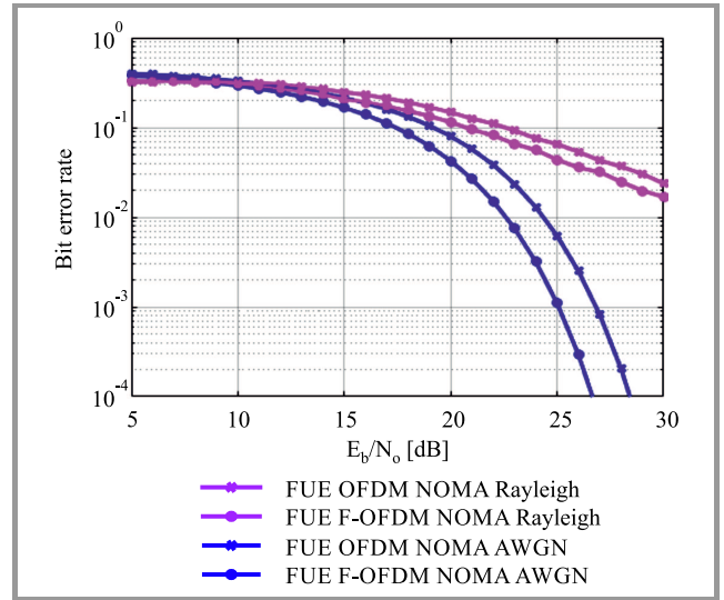
Fig. 14. The BER performance of FUE in uplink F-OFDM NOMA in AWGN and Rayleigh channel.
