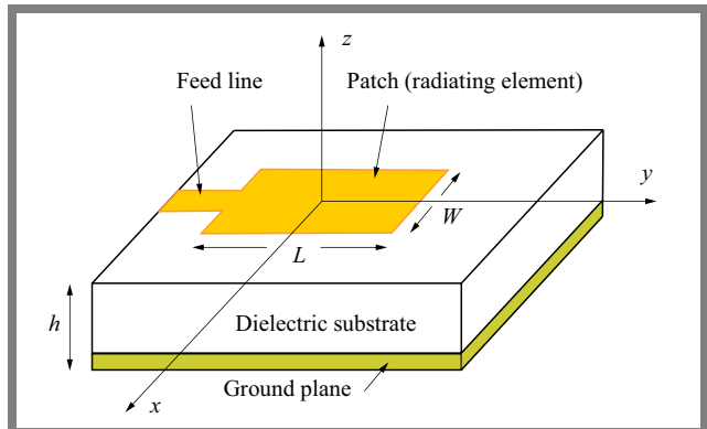
Fig. 1. Microstrip antenna.
